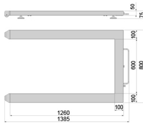
PWI: Abmessungen in mm
